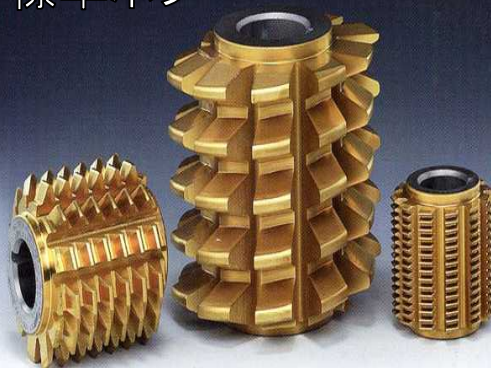
標準ホブ
